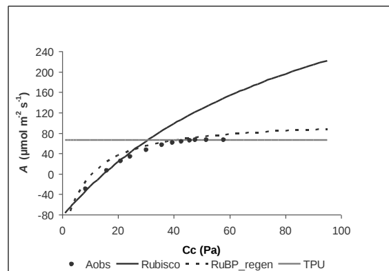
Figura 1. Curva di risposta della fotosintesi netta ( A ) alla pressione parziale della \text{CO}_2 nella RUBISCO ( C_c ); ( A_{\text{obs}} = valori di A osservati; \text{RuBP\_regen} = A limitata dalla disponibilità di Ribulosio 1,5 Bifosfato; \text{TPU} = A limitata dalla disponibilità dei trioso-fosfati).
