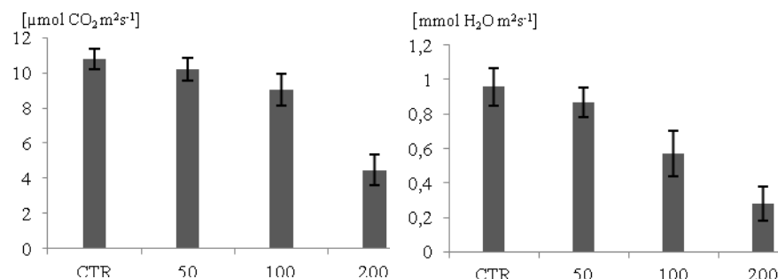
Fig. 1 – Confronto grafico fra i valori del tasso fotosintetico [ \mu\text{mol CO}_2 \text{ m}^{-2} \text{ s}^{-1} ], a sinistra, ed il tasso di traspirazione [ \text{mmol H}_2\text{O m}^{-2} \text{ s}^{-1} ], a destra, misurati nelle quattro differenti tesi sperimentali.
